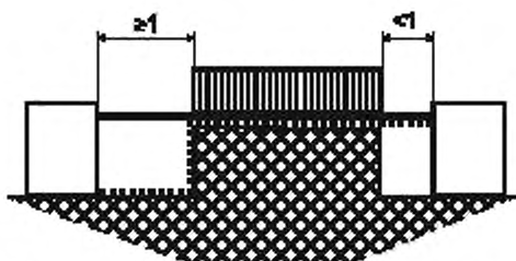
Рисунок А.1b — Зазор для ребра и бесклевого стыка с пазом
