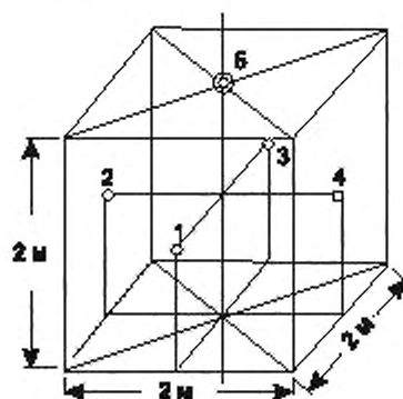
Рисунок I.3 — Точки измерения на кубической измерительной поверхности
