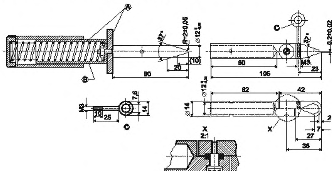
A — изоляционный материал; B — диаметр пружины; C — проушина
