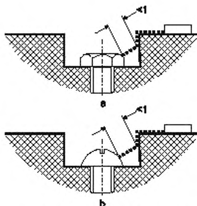
Рисунок A.1c — Зазор для бесклевого стыка и паза с расходящимися стенкам
