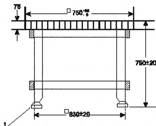
Рисунок I.1 — Испытательная стойка
