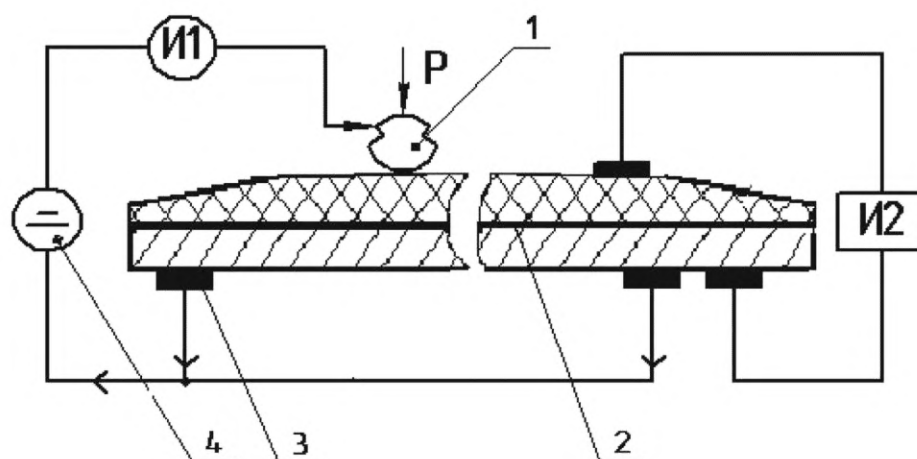
1 — отрезок контактного провода; 2 — вставка; 3 — медная пластина — электрод; 4 — источник постоянного тока; I1 — амперметр; I2 — милливольтметр; P — усилие прижатия
