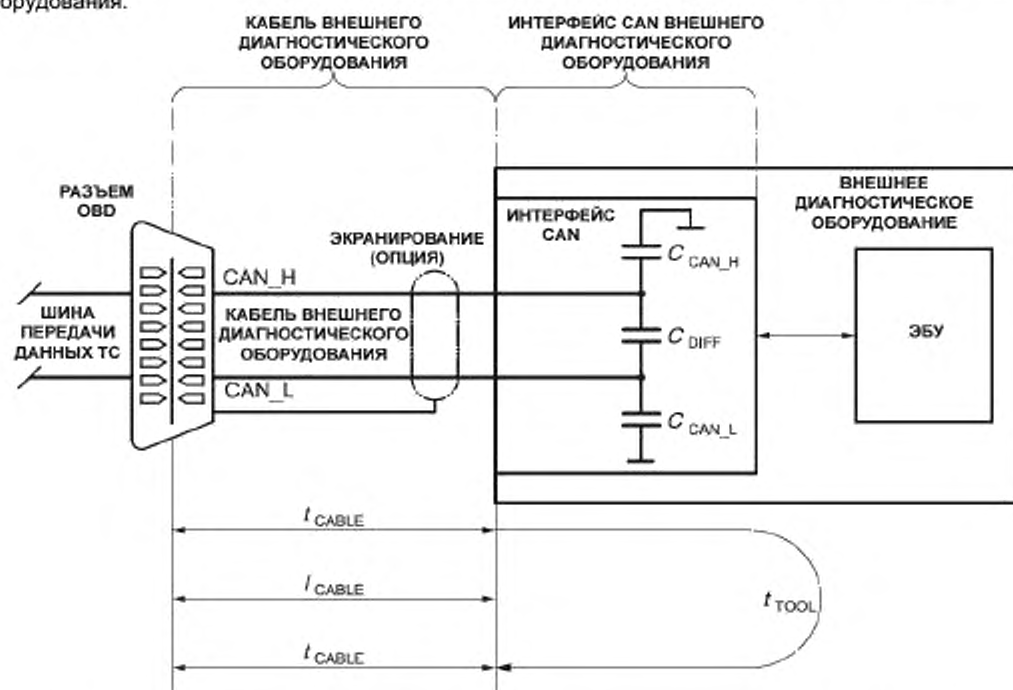
Рисунок 9 – Электротехнические параметры внешнего диагностического оборудования
