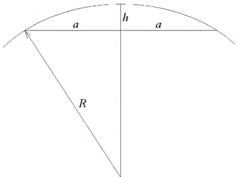
Рисунок 1 — Схема измерения радиуса кривой
