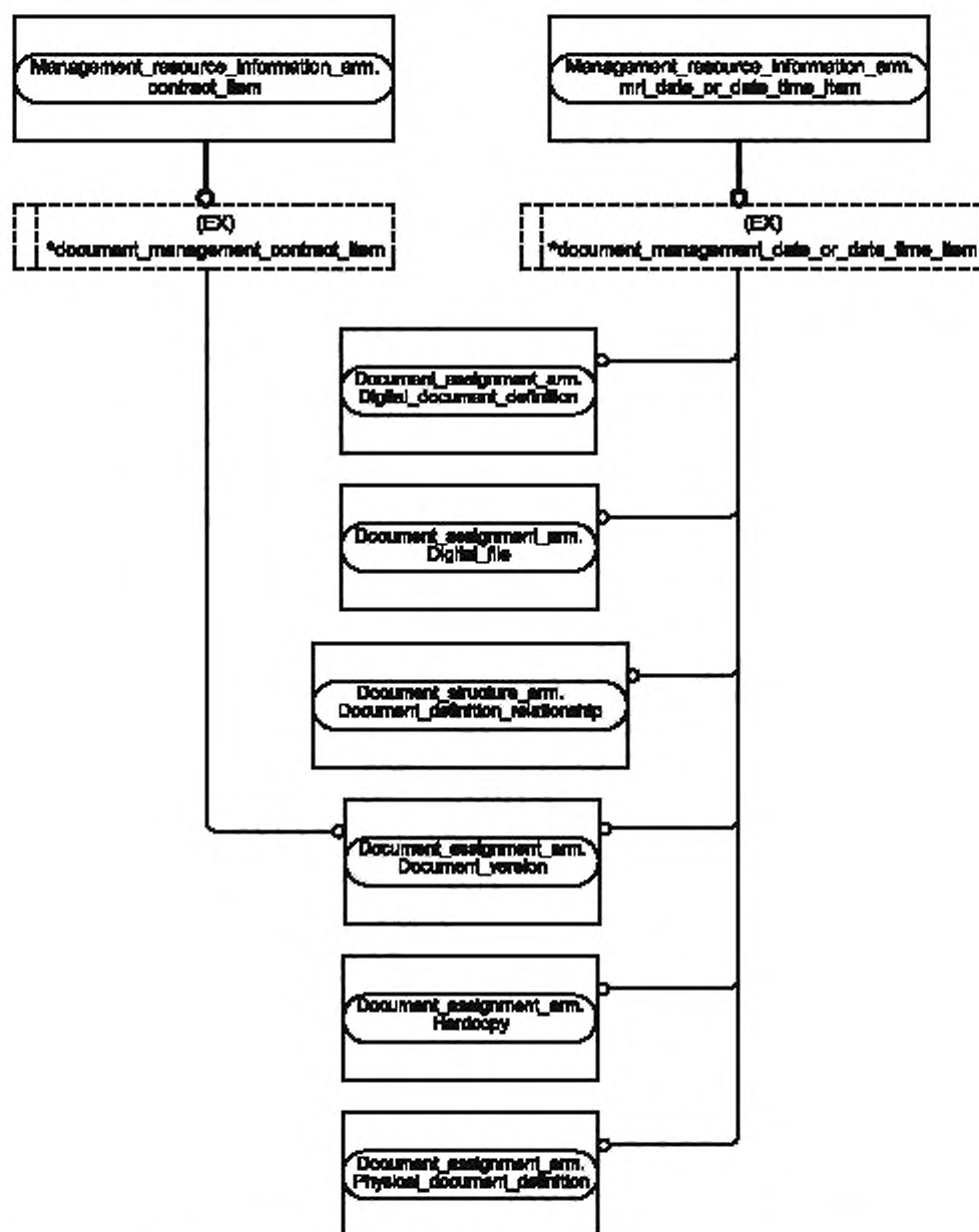
Рисунок С.3 — Представление ПЗМ на уровне объектов в формате EXPRESS-G (диаграмма 2 из 4)
