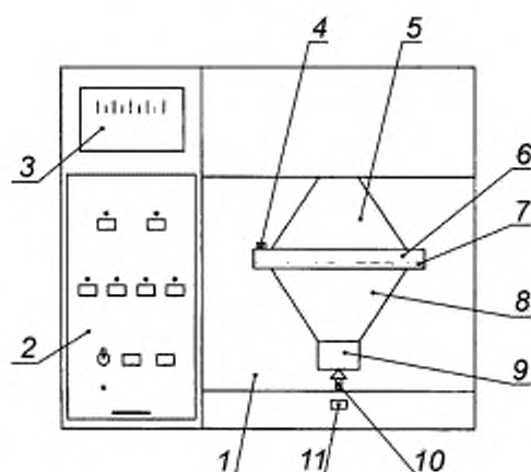
1 — корпус; 2 — блок электронный; 3 — тягомер; 4 — фиксатор; 5 — воронка верхняя; 6 — сито; 7 — устройство зажимное; 8 — воронка нижняя; 9 — ювета; 10 — упор; 11 — педаль
