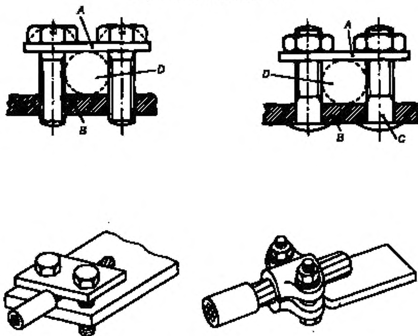
Рисунок D.3 — Штифтовые зажимы
