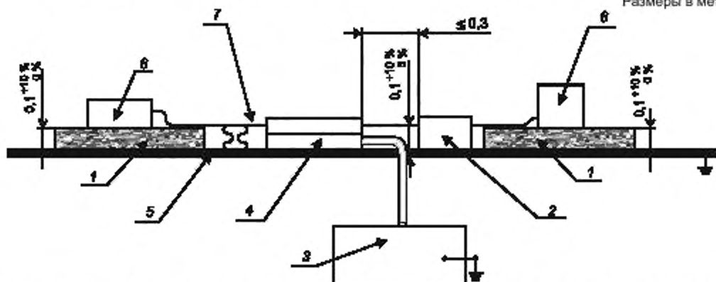
1 – изоляционная опора; 2 – развязывающее устройство; 3 – РЧ генератор; 4 – электромагнитные клещи; 5 – плата заземления; 6 – испытуемый аппарат (ИА); 7 – кабель ( 0,1 \text{ м} \leq \text{длина кабеля} \leq 0,3 \text{ м} ); 8 – вспомогательное оборудование.
