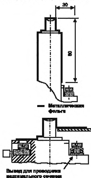
Рисунок R.2 – Оперативное пространство для нажимной кнопки
