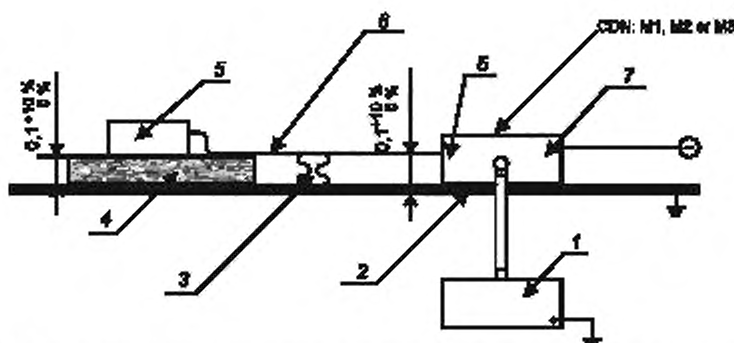
1 – генератор РЧ; 2 – плата заземления; 3 – изоляционная опора для кабелей; 4 – изоляционное основание; 5 – испытуемый аппарат (ИА); 6 – кабель ( 0,1 \text{ м} \leq \text{длина кабеля} \leq 0,3 \text{ м} ); 7 – сеть питания; CDN – развязывающий фильтр
