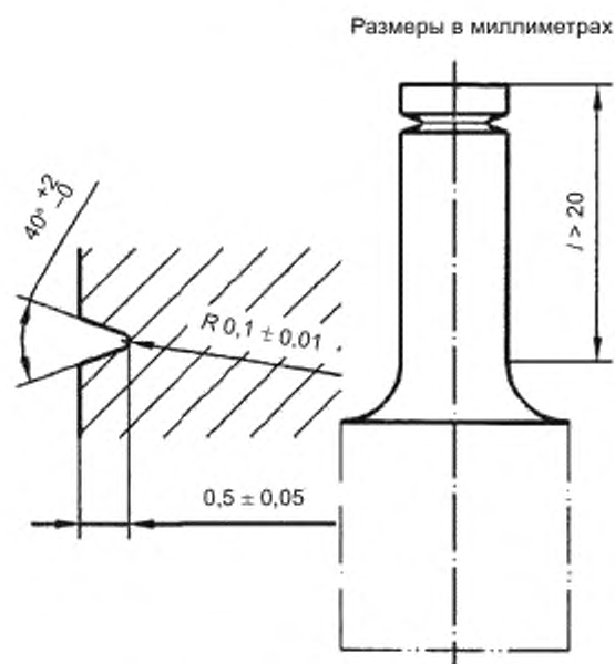
Рисунок 3 — Имплант кольцевой
