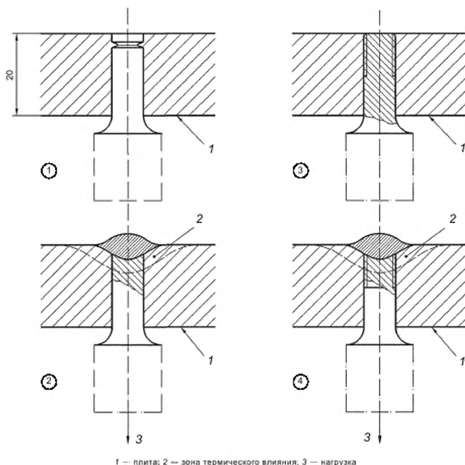
Рисунок 4 — Наплавка кольцевого и винтового импланта
