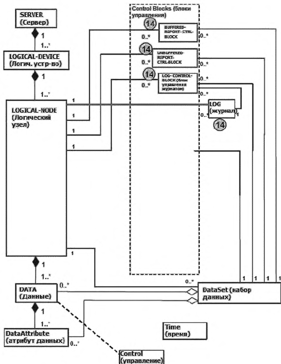
Рисунок В.1 – Концептуальная модель сервиса ACSI
