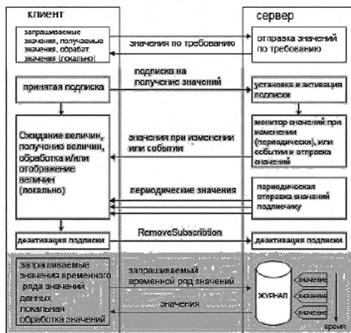
Рисунок 4 – Концепция модели мониторинга, регистрации и выдачи отчетов
