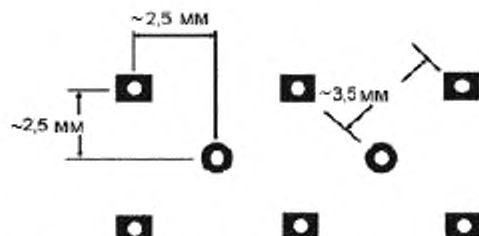
Единичный тест-купон волнового сопротивления Схема образца 1А
