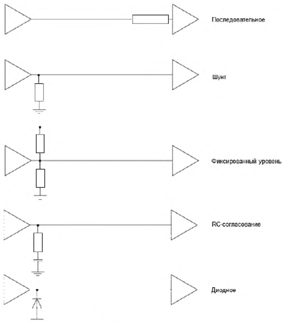
Рисунок 3 – Согласование нагрузок
