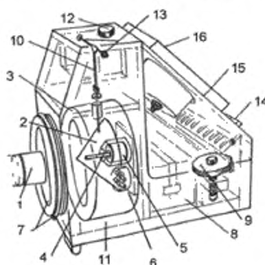
1 — преобразователь; 2 — полая коническая мишень; 3 — поглотитель; 4 — магнит для уравнивания радиационной силы; 5 — катушка для уравнивания радиационной силы; 6 — индикаторы нуля на светодиодах; 7 — мембрана с фланцем; 8 — свинцово-кислотная батарея; 9 — установка нуля; 10 — подвеска мишени; 11 — камера с водой; 12 — крышка с фильтром; 13 — цапфы на камнях; 14 — переключатель диапазонов, электронный блок, показывающее устройство
