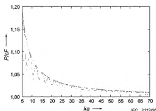
Рисунок Е.1 — Зависимость P/cF от ka (осциллирующая линия) с аппроксимацией «по пикам» (сплошная линия) и центральной (по половинным значениям) линии (пунктирная линия), представляющей поправочный коэффициент scat
