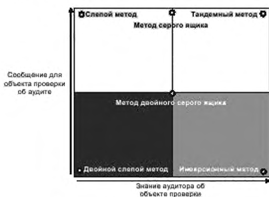
Рисунок 1 – Виды тестирования
