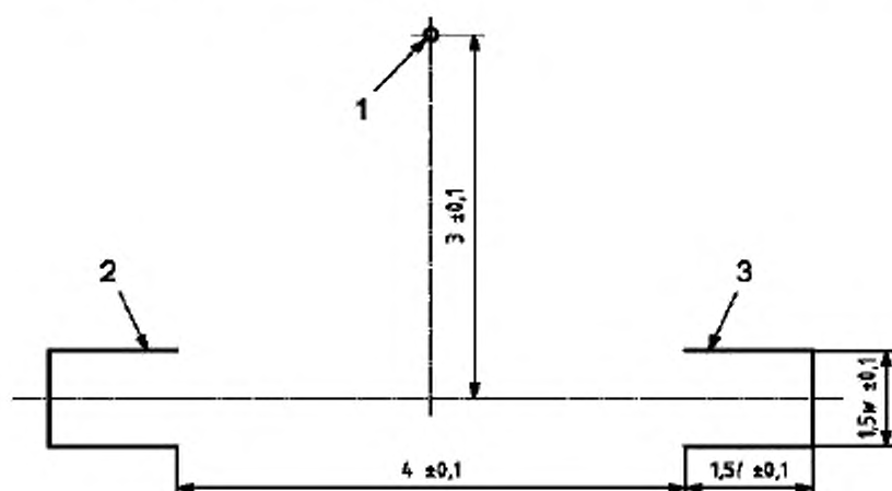
Рисунок 1 — Испытательная трасса
