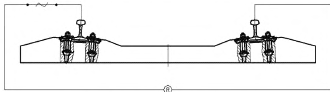
Рисунок 6 — Схема измерения электрического сопротивления
