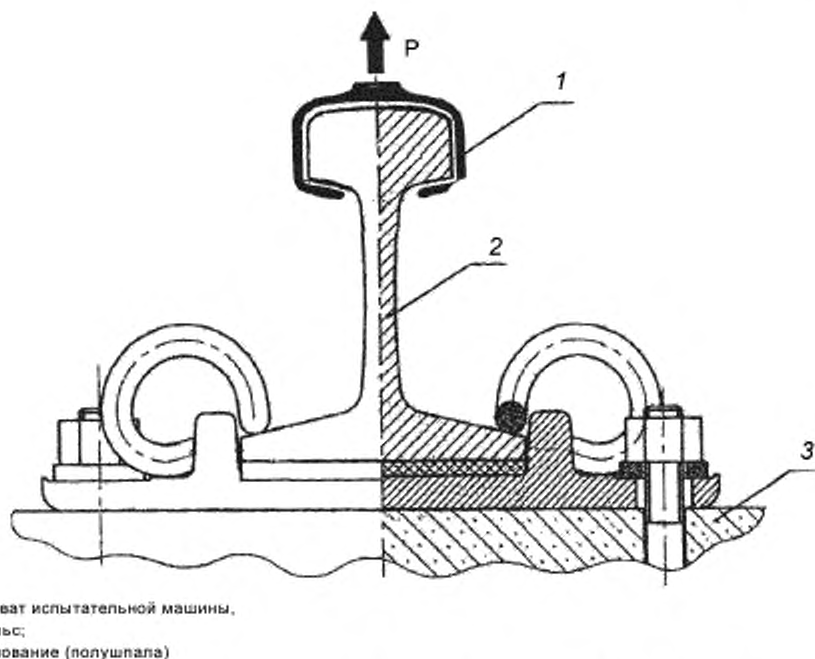
Рисунок 3 — Схема нагружения узла рельсового скрепления (условного) для определения усилия монтажного прижатия рельса к шпалам
