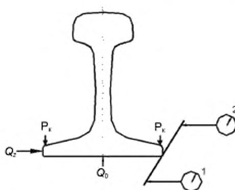
Рисунок 4 — Схема нагружения узла рельсового скрепления для определения его вертикальной жесткости D_{cy}
