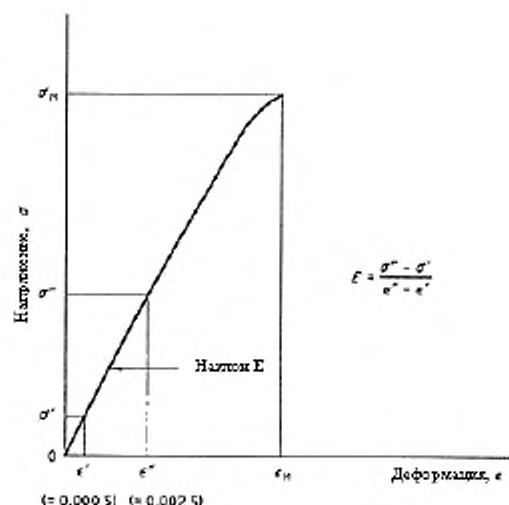
Рисунок 2 — Диаграмма напряжение-деформация
