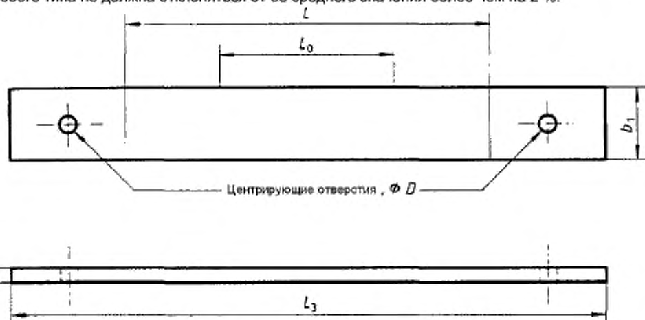
Рисунок 5 – Образец типа 2
