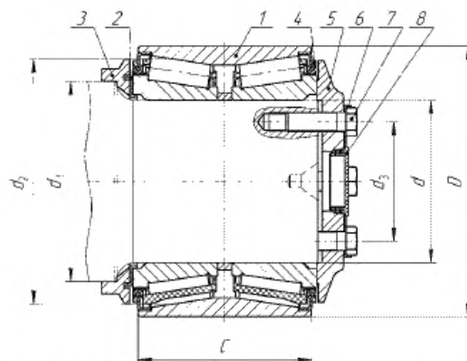
1 – базовый подшипник; 2 – полимерная прокладка; 3 – упорное кольцо; 4 – уплотнение; 5 – передняя крышка; 6 – стопорная шайба; 7 – болт торцевого крепления; 8 – заглушка
