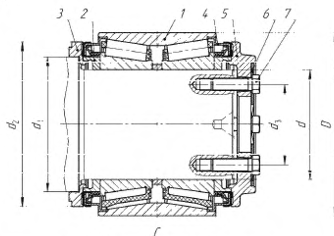
1 – базовый подшипник; 2 – компенсационное кольцо; 3 – упорное кольцо; 4 – уплотнение; 5 – передняя крышка; 6 – стопорная шайба; 7 – болт торцевого крепления
