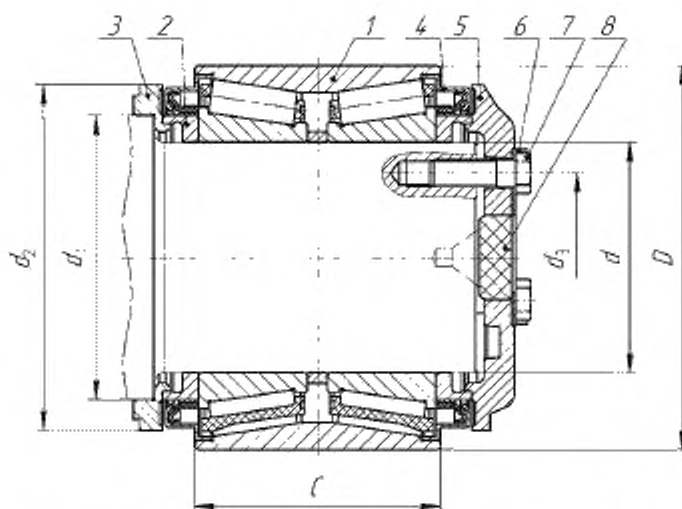
1 – базовый подшипник; 2 – компенсационное кольцо; 3 – упорное кольцо; 4 – уплотнение; 5 – передняя крышка; 6 – стопорная шайба; 7 – болт торцевого крепления; 8 – заглушка
