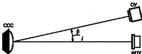
ОУ — осветительное устройство; ФПУ — фотоприемное устройство; \beta — угол падения луча ОУ на CCC (угол засветки CCC); l — расстояние от CCC до ФПУ
