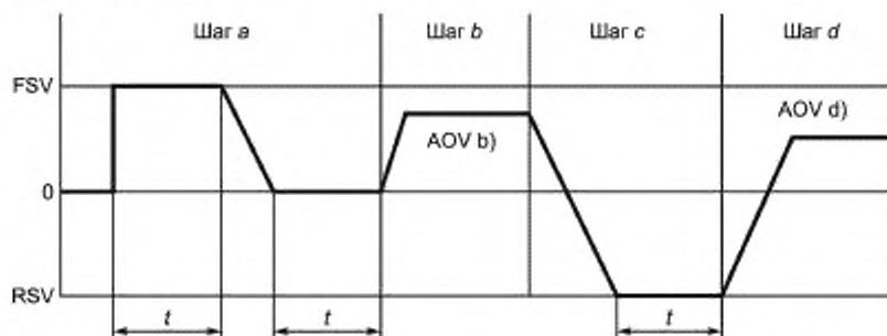
Рисунок 13 — Последовательная схема для теста остаточной намагниченности
