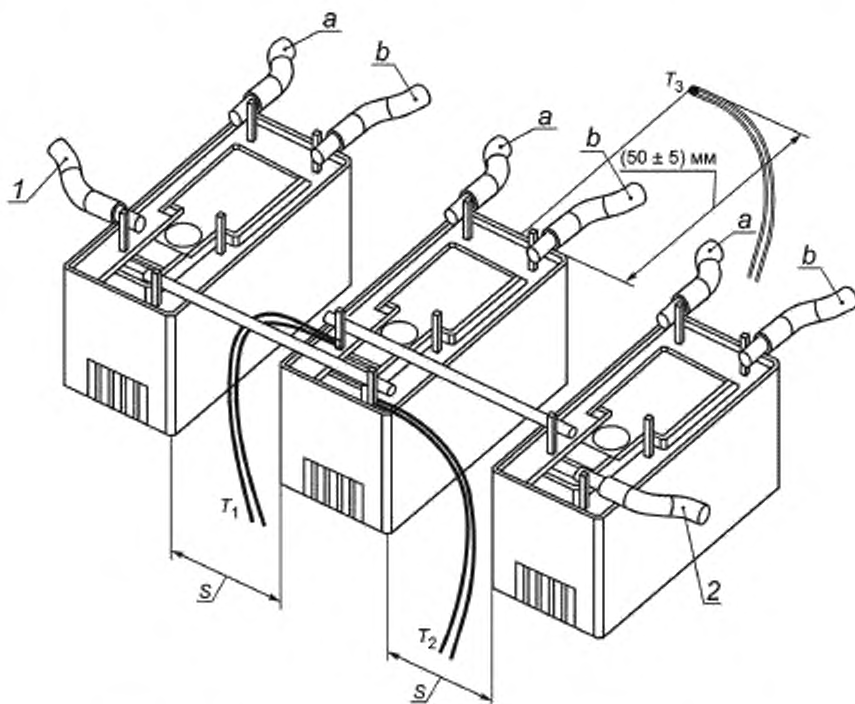
1, 2 — клеммы контактов; T_1 , T_2 , T_3 — термодатчики; a, b — клеммы катушек, S — расстояние монтажа
