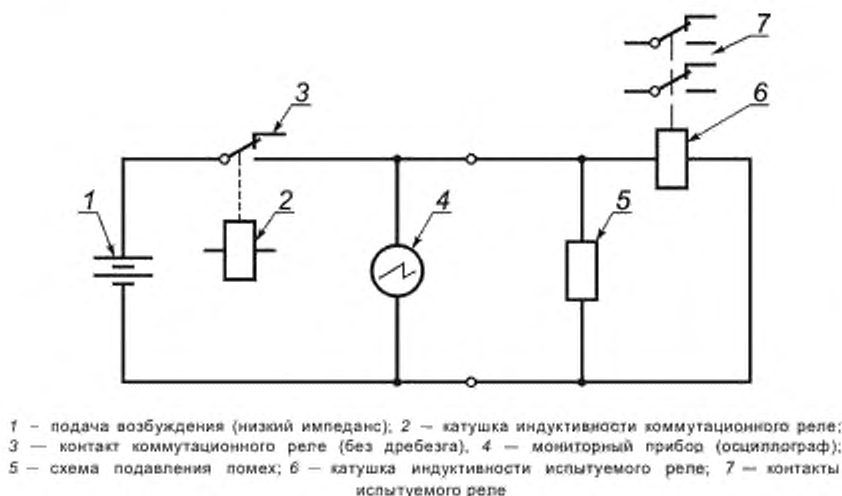
Рисунок 1 — Типичная схема измерения подавления переходных помех катушки
