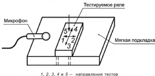
Рисунок 14 — Установка для теста излучения акустических шумов
