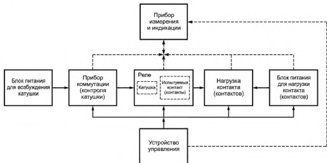
Рисунок С.2 — Функциональная блок-схема
