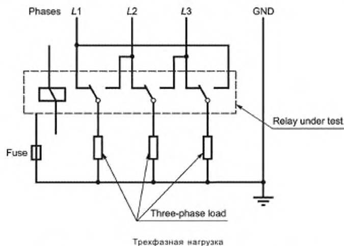
Рисунок 10 — Тестовая схема для переноса нагрузки
