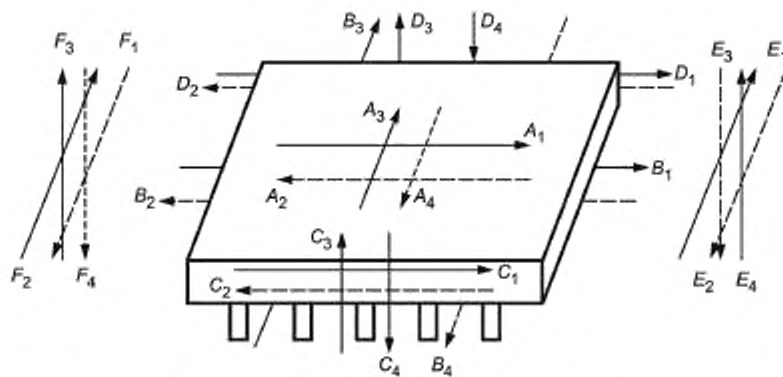
Направления тестового тока с A_1 по F_4
