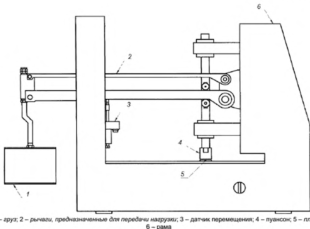
Рисунок 1 – Устройство для приложения постоянной нагрузки к образцу для испытаний
