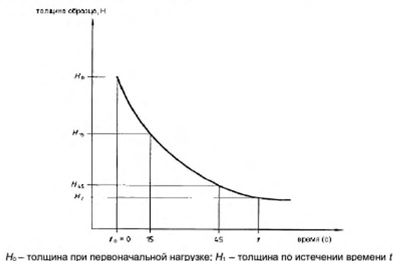
Рисунок 5 — Стандартная кривая текучести, определенная методом 1
