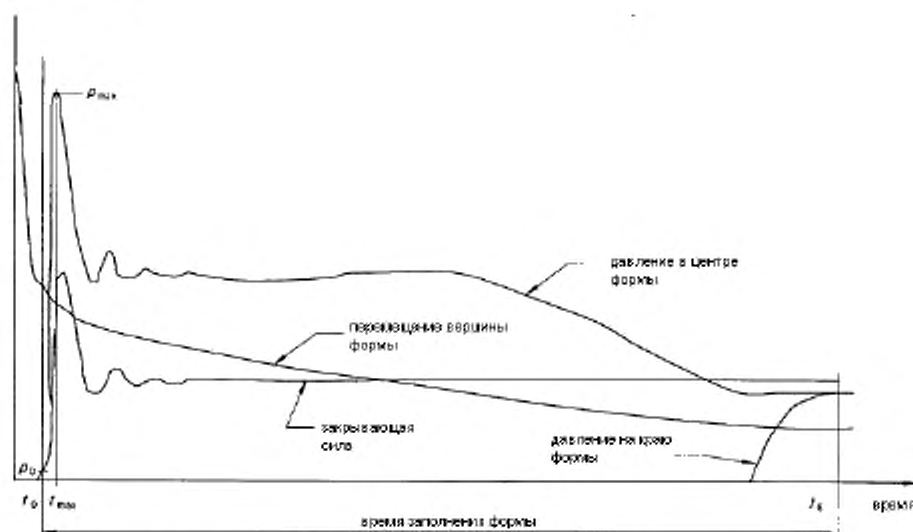
Рисунок 6 – Стандартные кривые, определенные методом 2
