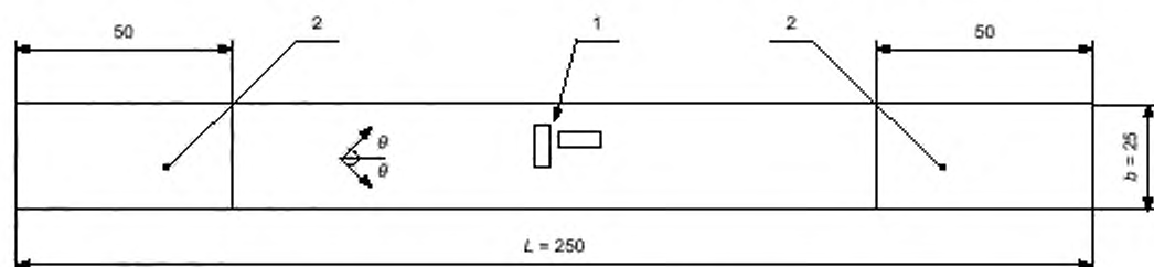
1 – датчики деформации; 2 – концевые участки; \theta – угол ориентации волокон
