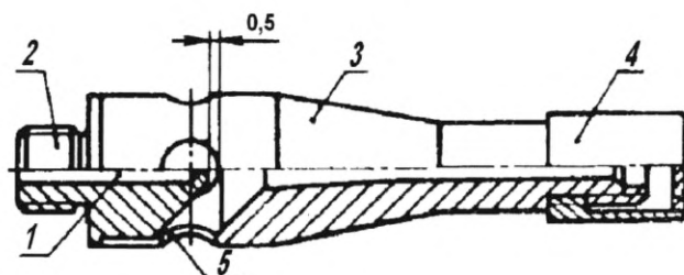
1 — дроссельная трубка; 2 — газовое сопло; 3 — трубка горелки; 4 — стабилизатор пламени; 5 — выемка
