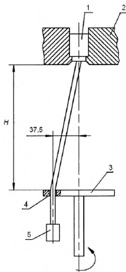
1 — испытуемый зажим; 2 — крепление; 3 — плата; 4 — втулка; 5 — груз
