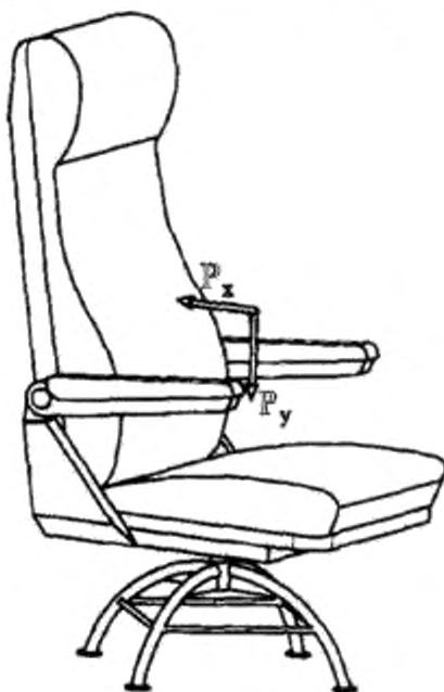
Рисунок В.1 Схема нагружения
