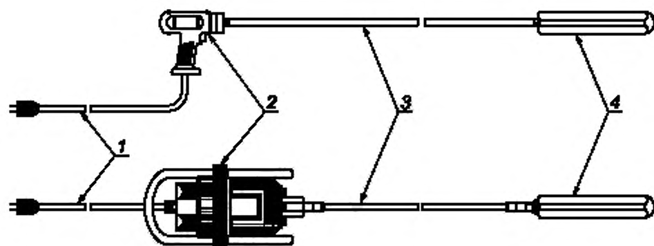
1 — кабель электропитания; 2 — блок, содержащий сетевой выключатель и электродвигатель; 3 — гибкий вал, 4 — вибронаконечник
