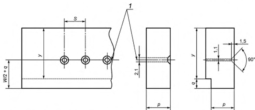
а) Пластины для пресс-формы к рисунку 1
