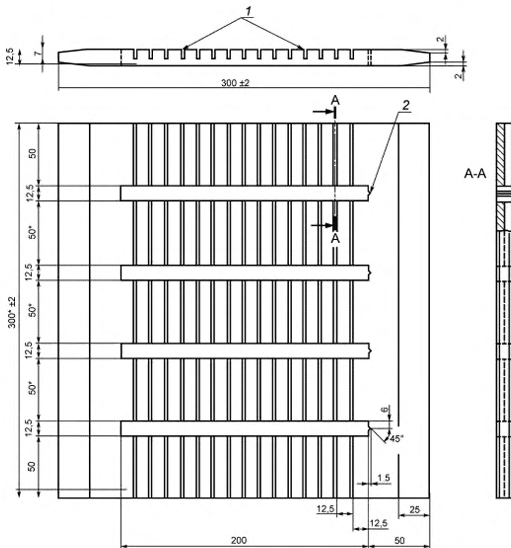
1—15 прорезей шириной (1,6 \pm 0,1) мм; 2 — идентификационный номер
