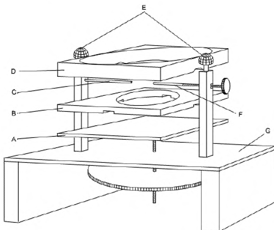
A — регулируемая платформа; B — нижняя часть маски (см. деталь A, на рисунке 103 а); C — фиксированный электрод; D — верхняя часть маски (см. деталь B, на рисунке 103 а); E — зажимы; F — подвижный электрод; G — основание пластины.
