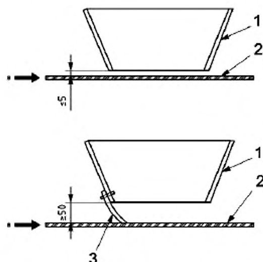
1 — стальной бункер, лоток; 2 — лента конвейера; 3 — резиновый скат; а) — направление движения ленты конвейера
