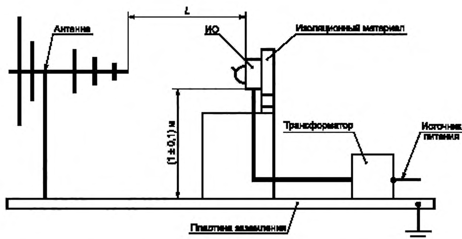
Рисунок 25 — Испытательная установка излучения радиопомех
