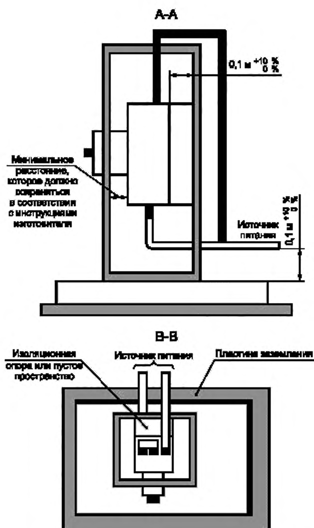
Рисунок 3б — Сечения А-А и В-В
