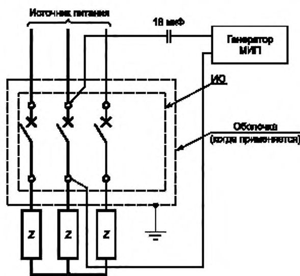
Рисунок 22 — Испытательная цепь для проверки влияния импульсов напряжения/тока на главную цепь. Трехфазная конфигурация
