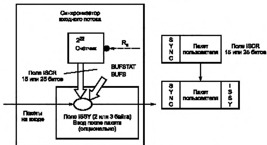
Рисунок А.1 — Блок-схема синхронизатора входного потока
