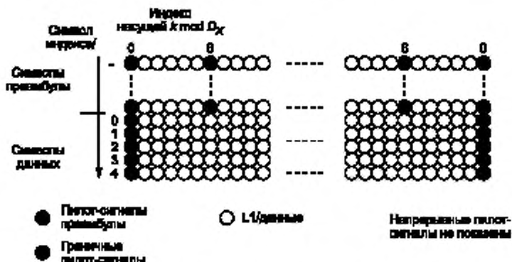
Рисунок 41 — Расположение граничных пилот-сигналов в спектре OFDM сигнала
