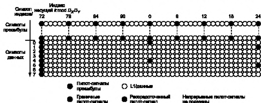
Рисунок Е.8 — Рассредоточенный пилот-сигнал для GI 1/128 с низкочастотной границей k \bmod D_X D_Y = 72
