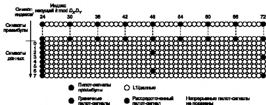
Рисунок Е.6 — Рассредоточенный пилот-сигнал для GI 1/128 с низкочастотной границей k \bmod D_X D_Y = 24
