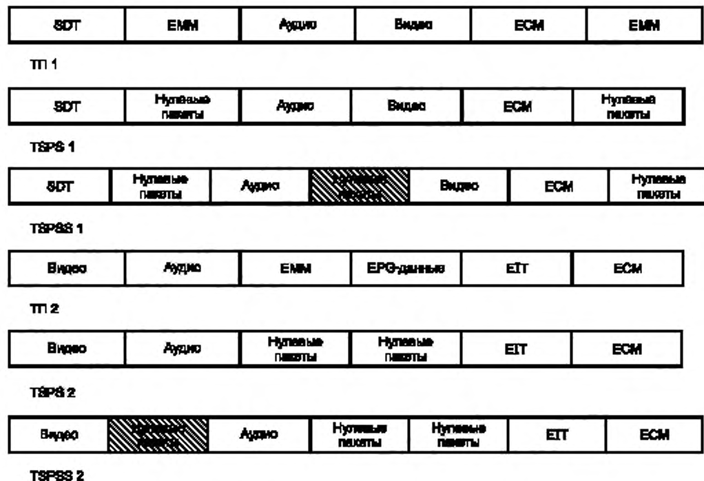
Рисунок Б.3 — Пример вставки нулевых пакетов на два TS / TSPS
