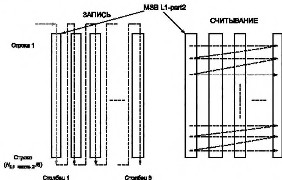
Рисунок 30 — Схема перемежителя битов данных L1-part2 (16QAM)
