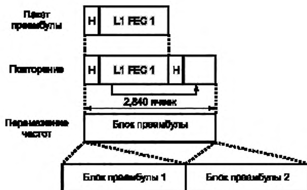
Рисунок 28 — Распределение L1 FECFrame на блоки L1 (блоки преамбулы)
