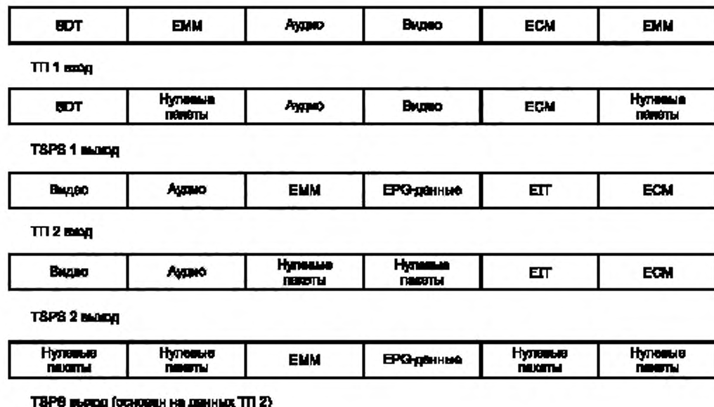
Рисунок Б.2 — Пример формирования двух TSPS и формирования TSPSC из двух входных TS
