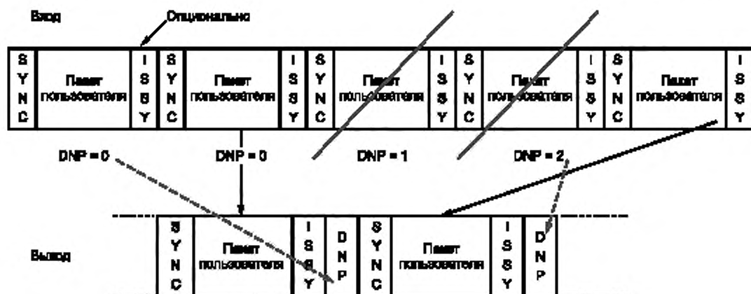
Рисунок 6 — Схема удаления нулевых пакетов
