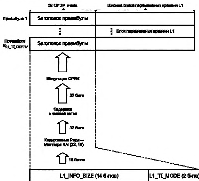
Рисунок 23 — Формирование заголовка преамбулы и полей сигнализации
