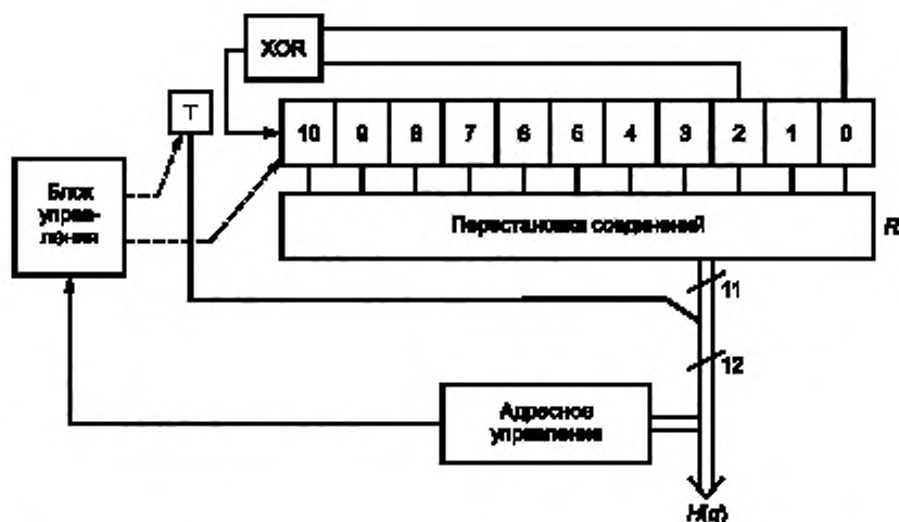
Рисунок 40 — Блок-схема алгоритма формирования функции перестановки переключателя частоты режима 4К
