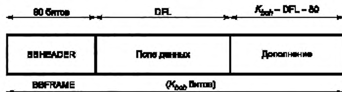
Рисунок 12 — Формат кадра BBFrame на выходе адаптера потока
