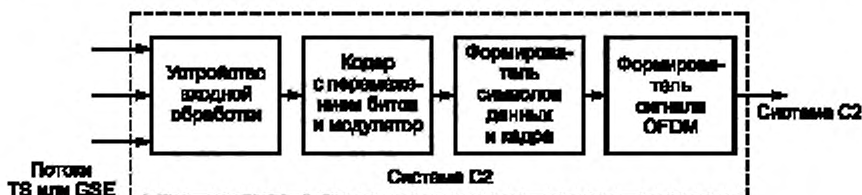
Рисунок 1 — Обобщенная модель формирования Системы C2
