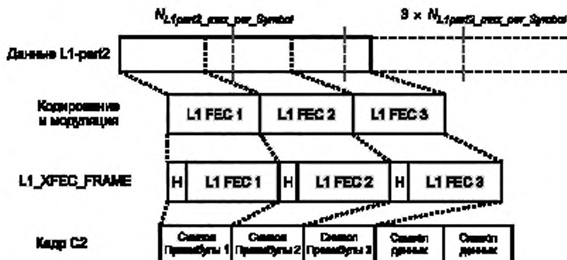
Рисунок 27 — Длина кодированных данных
