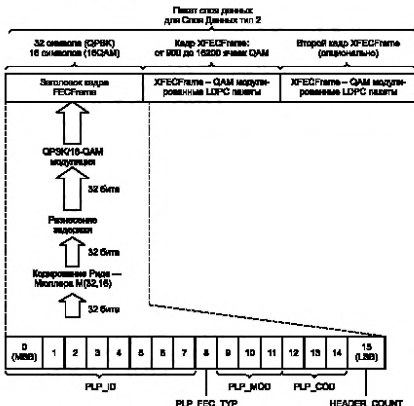
Рисунок 19 — Пакет Слая Данных Тип 2, состоящий из заголовка FECFrame и следующих за ним пакетов XFECFrame
