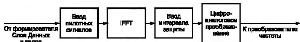
Рисунок 5 — Блок-схема подсистемы формирования сигнала OFDM
