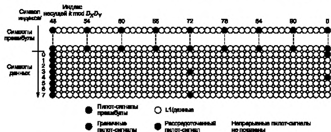
Рисунок Е.7 — Рассредоточенный пилот-сигнал для GI 1/128 с низкочастотной границей k \bmod D_X D_Y = 48
