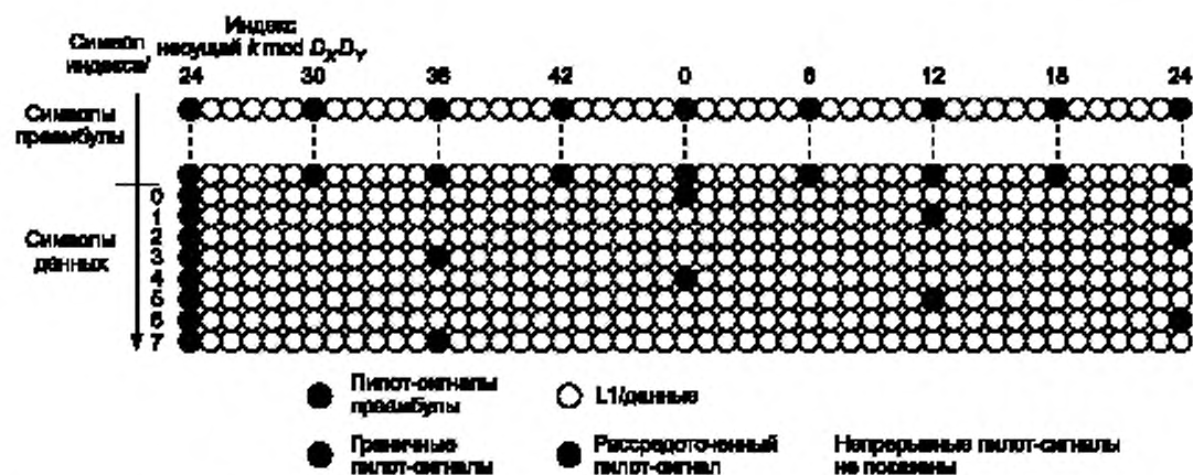
Рисунок E.3 — Рассредоточенный пилот-сигнал для GI 1/64 с низкочастотной границей k \bmod D_x D_y = 24
