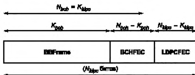
Рисунок 14 — Формат данных перед операцией перемежения битов ( N_{ldpc} = 64\,800 битов для нормального кадра FECFrame, N_{ldpc} = 16\,200 битов для короткого FECFrame)
