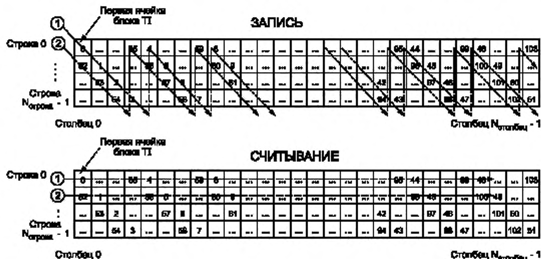
Рисунок 32 — Перемеживание времени данных сигнализации L1 ( N_{MOD\_TOTAL} = 208 , N_{LI\_TI\_DEPTH} = 4 )
