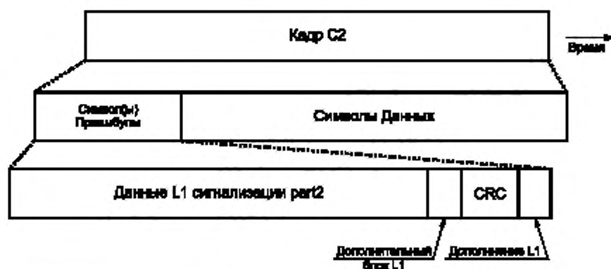
Рисунок 22 — Структура данных сигнализации L1-part2
