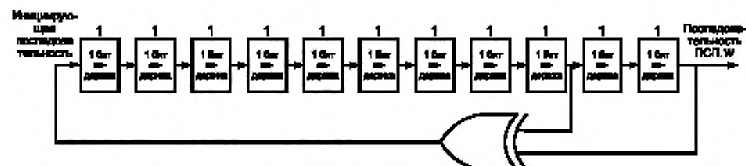
Рисунок 34 — Формирование псевдослучайной последовательности
