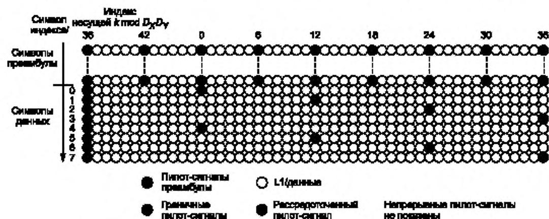
Рисунок E.4 — Рассредоточенный пилот-сигнал для GI 1/64 с низкочастотной границей k \bmod D_x D_y = 36
