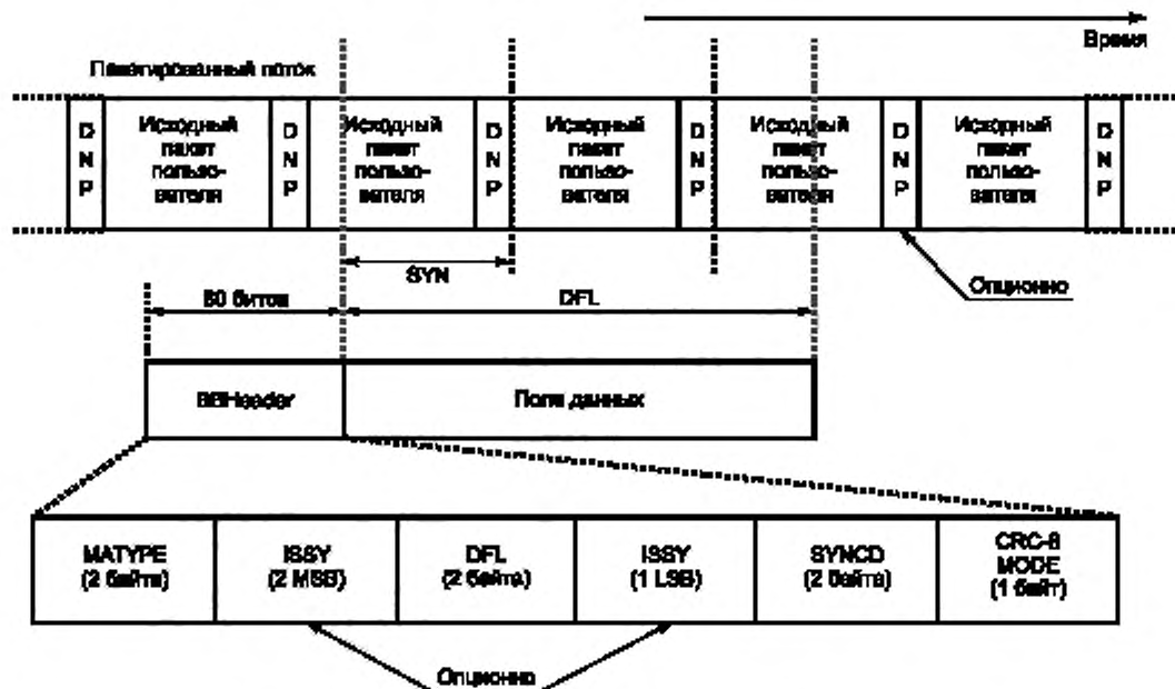
Рисунок 10 — Формат потока TS на выходе адаптера режима HEM
