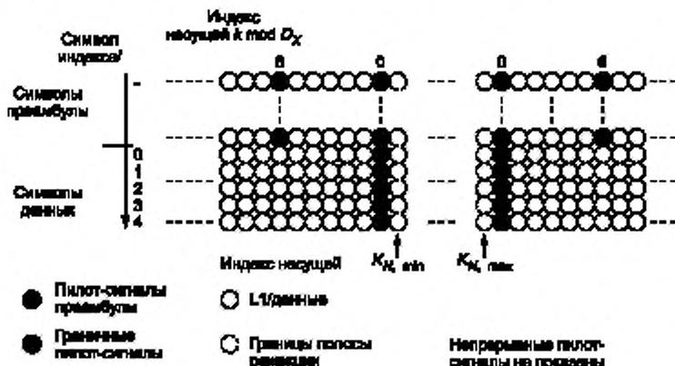
Рисунок 42 — Расположение граничных пилот-сигналов на границах полосы режекции
