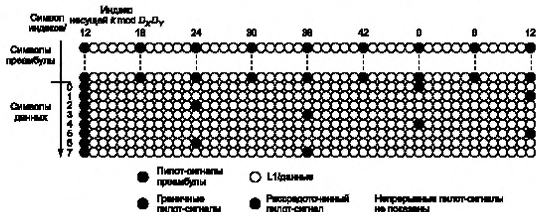
Рисунок Е.2 — Рассредоточенный пилот-сигнал для G_I = 1/64 с низкочастотной границей k \bmod D_x D_y = 12
