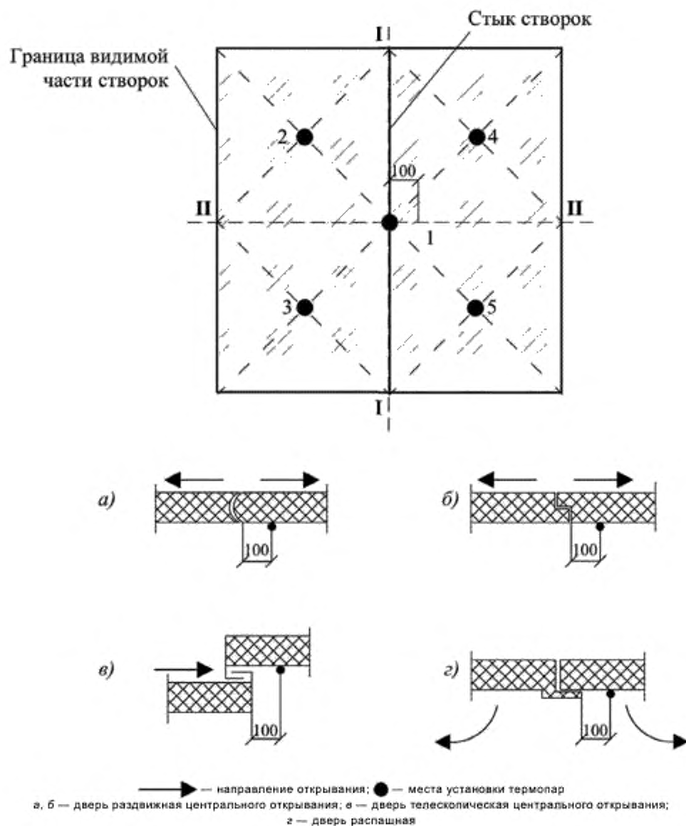
Рисунок А.4 — Схема установки термодатчиков на необогреваемой поверхности двухстворчатой двери
