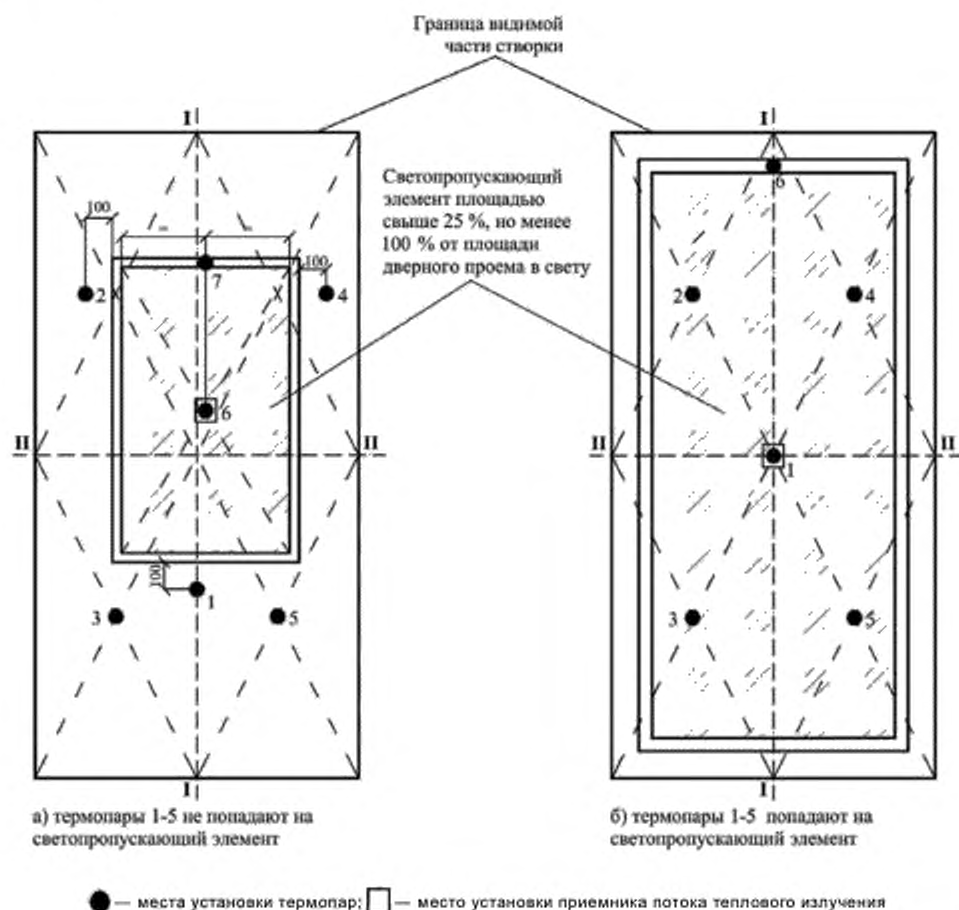
Рисунок А.3 — Схема установки термодатчиков и приемника потока теплового излучения на необогреваемой поверхности створки одностворчатой распашной и горизонтально-раздвижной двери бокового открывания со светопроницающим элементом створки свыше 25 %, но менее 100 % от площади проема в свету
