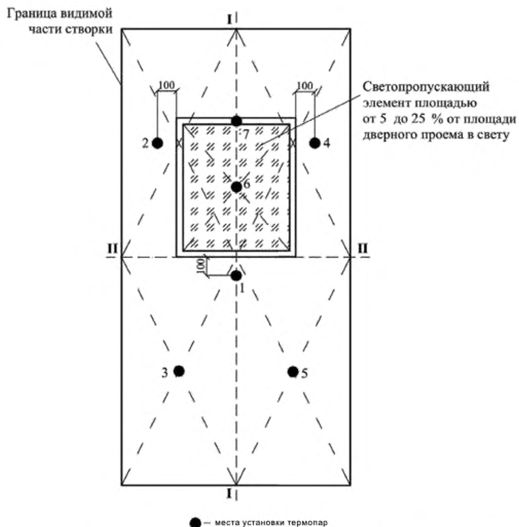
Рисунок А.2 — Схема установки термодатчиков на необогреваемой поверхности створки односторонней распашной и горизонтально-раздвижной двери бокового открывания со светопропускающим элементом створки свыше 5 % до 25 % от площади дверного проема в свету
