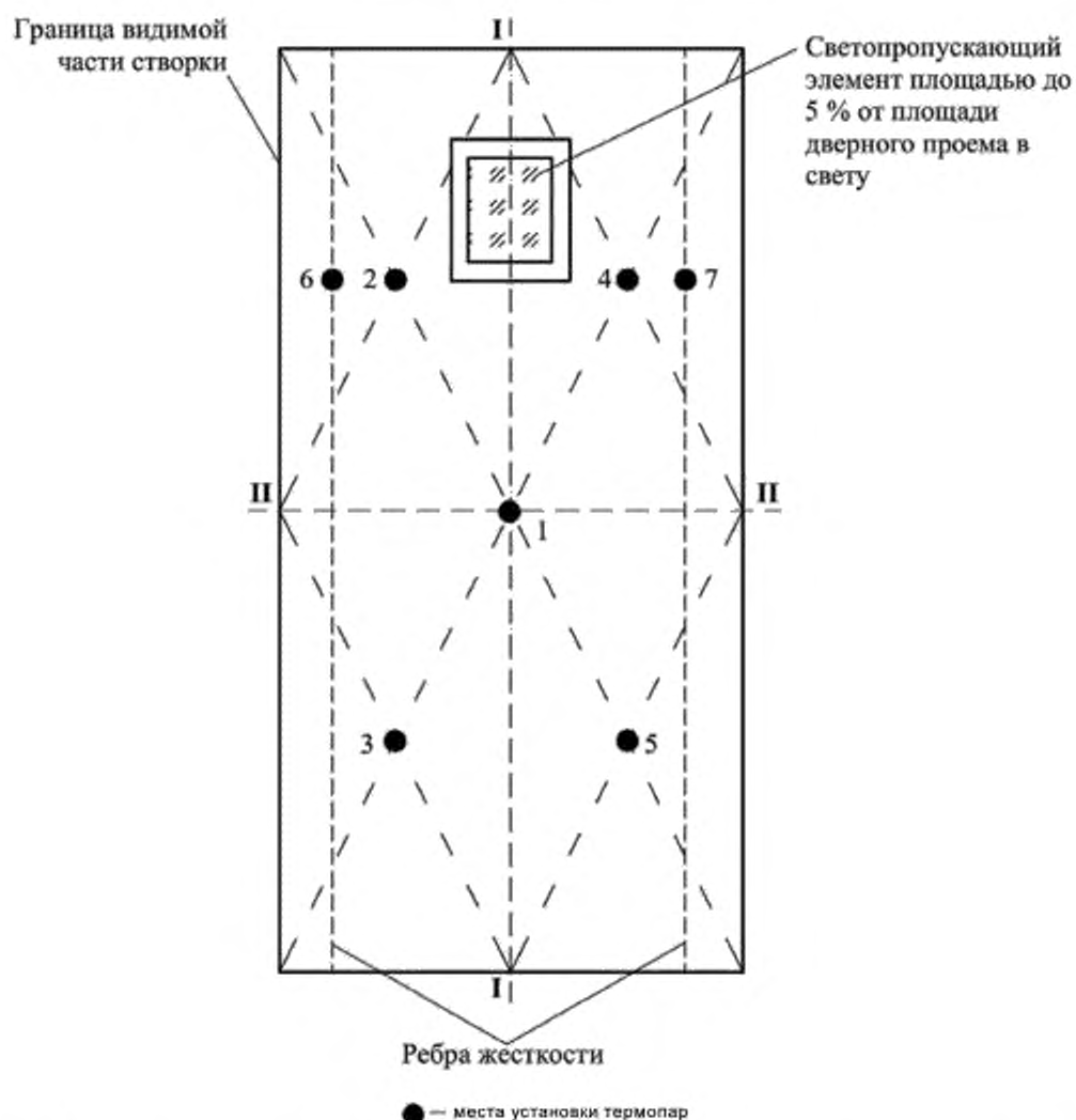
Рисунок А.1 — Схема установки термопар на необогреваемой поверхности створки одностворчатой распашной и сплошной горизонтально-раздвижной двери бокового открывания и со светопропускающим элементом створки до 5 % от площади дверного проема в свету
