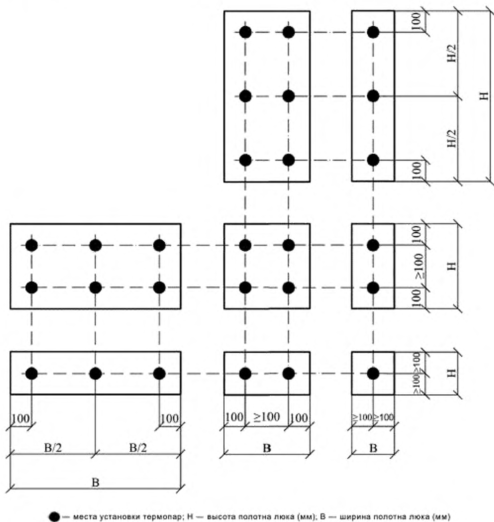
Рисунок А.5 — Схемы установки термодатчиков на необогреваемой поверхности люков площадью полотна, не превышающей 0,25 \text{ м}^2
