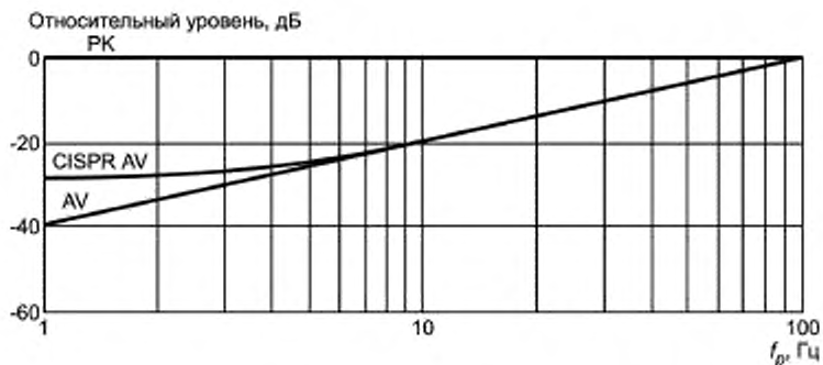
Рисунок С.2 — Весовая функция импульса 10 мс при детектировании пиковым детектором «PK», детектором средних значений при учете пиковых значений «CISPR AV» и детектором средних значений без учета пиковых значений «AV» для постоянной времени прибора 100 мс
