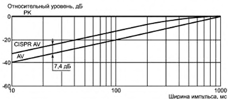
Рисунок С.3 — Пример весовых функций (импульс 1 Гц) при детектировании пиковым детектором «PK» и детектором средних значений «AV» относительно ширины импульсов для постоянной времени прибора 160 мс
