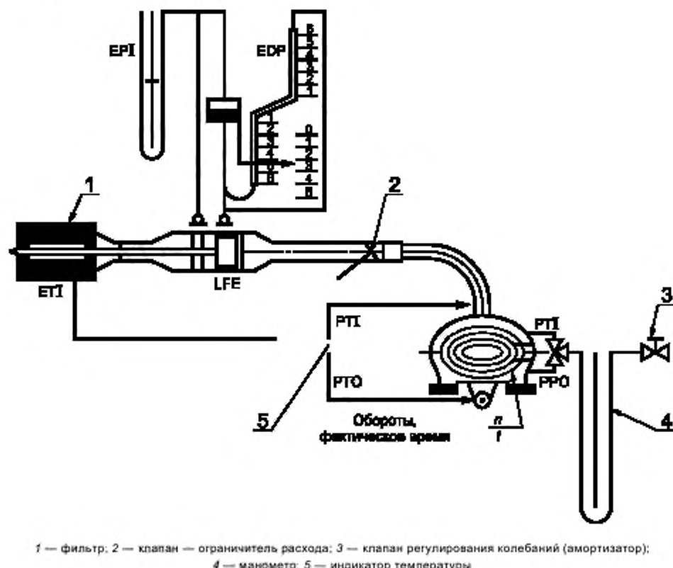
Рисунок Г.11 — Порядок соединения приборов для калибровки PDP-CVS
