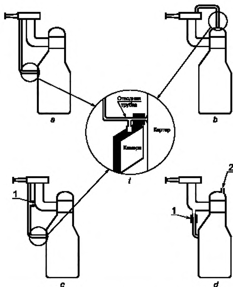
i — регулирующий клапан; 2 — вентиляционное отверстие; a — прямая рециркуляция при слабом разрежении; b — непряная рециркуляция при слабом разрежении; c — прямая двухканальная рециркуляция; d — вентиляция картера с применением регулирующего клапана (камера должна быть присоединена к вентиляционному отверстию); i — соединение отводной трубки и камеры
