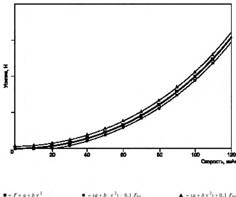
Рисунок Г.4 — График нагрузок, поглощенных динамометрическим стендом
