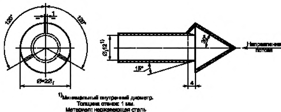
Рисунок Г.7 — Схема пробоотборника вредных частиц
