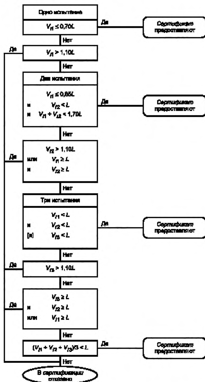
Рисунок 1 — Схема проведения сертификационных испытаний типа I
