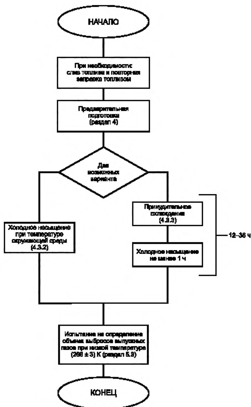
Рисунок К.1 — Процедура испытаний при низкой температуре окружающей среды
