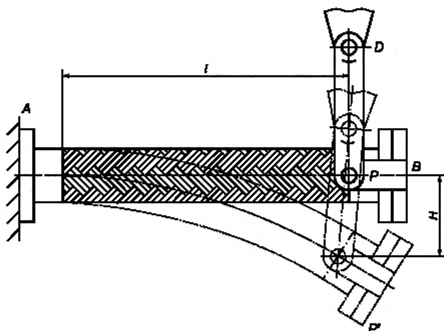
Рисунок 2 — Монтаж гибкого шланга в приспособление
