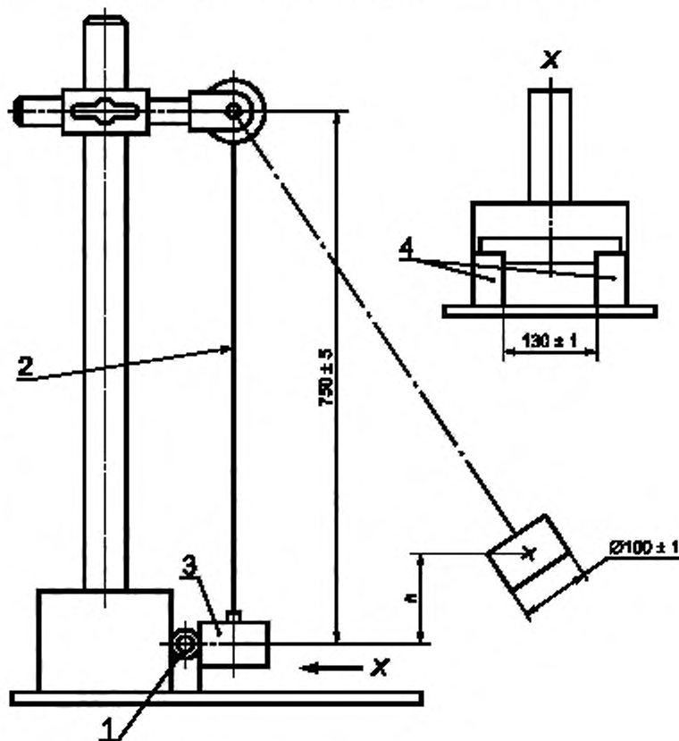
1 — газовый шланг; 2 — маятник; 3 — качающийся груз; 4 — опора шланга
