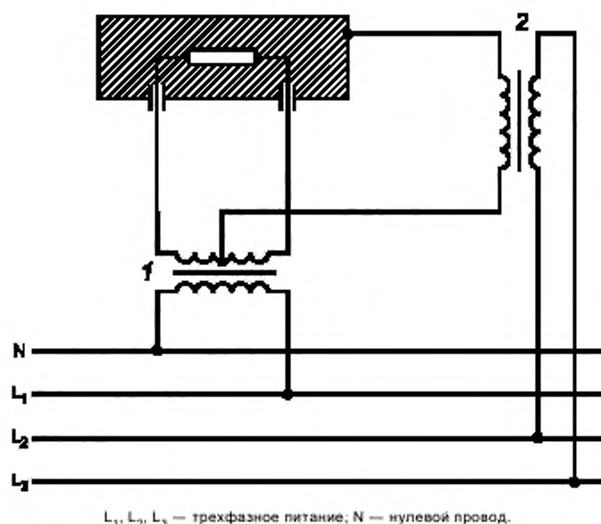
1 — разделительный трансформатор; 2 — повышающий трансформатор
