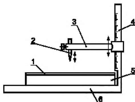
Рисунок А.2 — Испытательное устройство для объемных нетканых полотен толщиной более 20 мм
