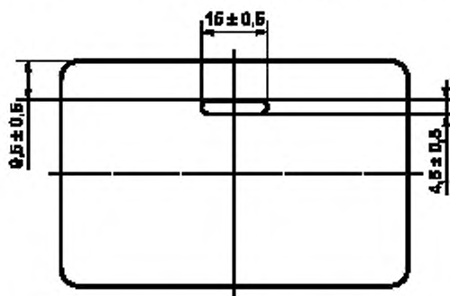
Рисунок В.2 — Щелевое отверстие для пейзажной ориентации
