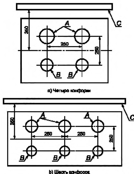
Рисунок 101 — Расположение для испытания на нагрев конфорочной панели
