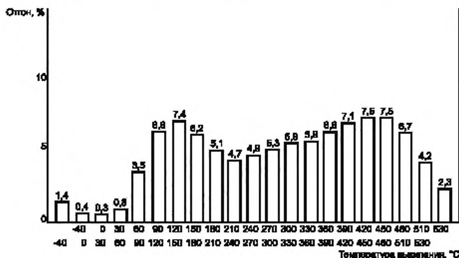
Рисунок А.1 — Диаграмма кривой распределения фракций по температурам выкипания жидкого композитного топлива
