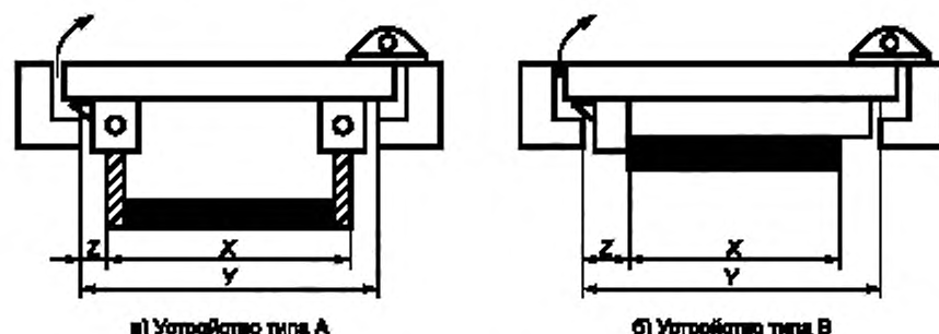
X — оптимальная длина штанги; Y — ширина полотна дверного блока в закрытом положении; Z — расстояние от штанги до коробки дверного блока
