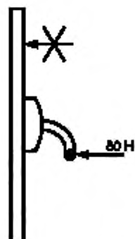
Рисунок В.5 — Схема приложения усилия для вывода засова из запорной планки устройства «Антипаника» для дверей эвакуационных выходов
