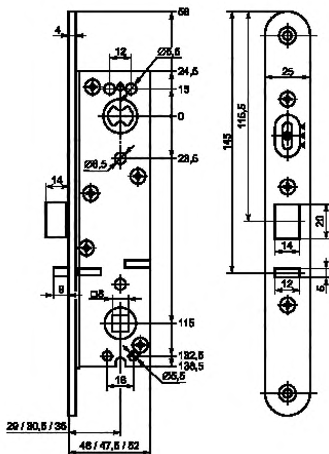
Рисунок А.5 — Пример замка электромеханического безключевого устройства «Антипаника» для дверей эвакуационных выходов
