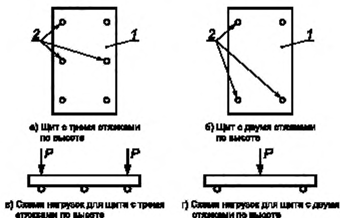
1 — щит; 2 — опора
