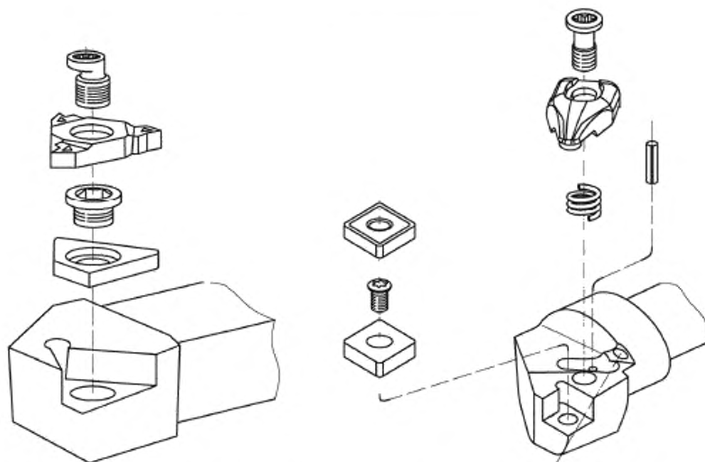
Рисунок Е.15 — Зажим эксцентриковым винтом
