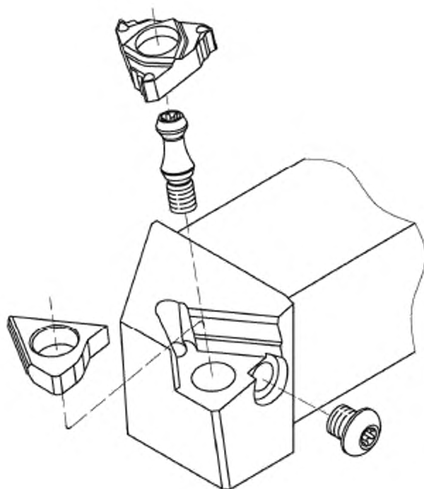
Рисунок Е.14 — Зажим отклонением винта
