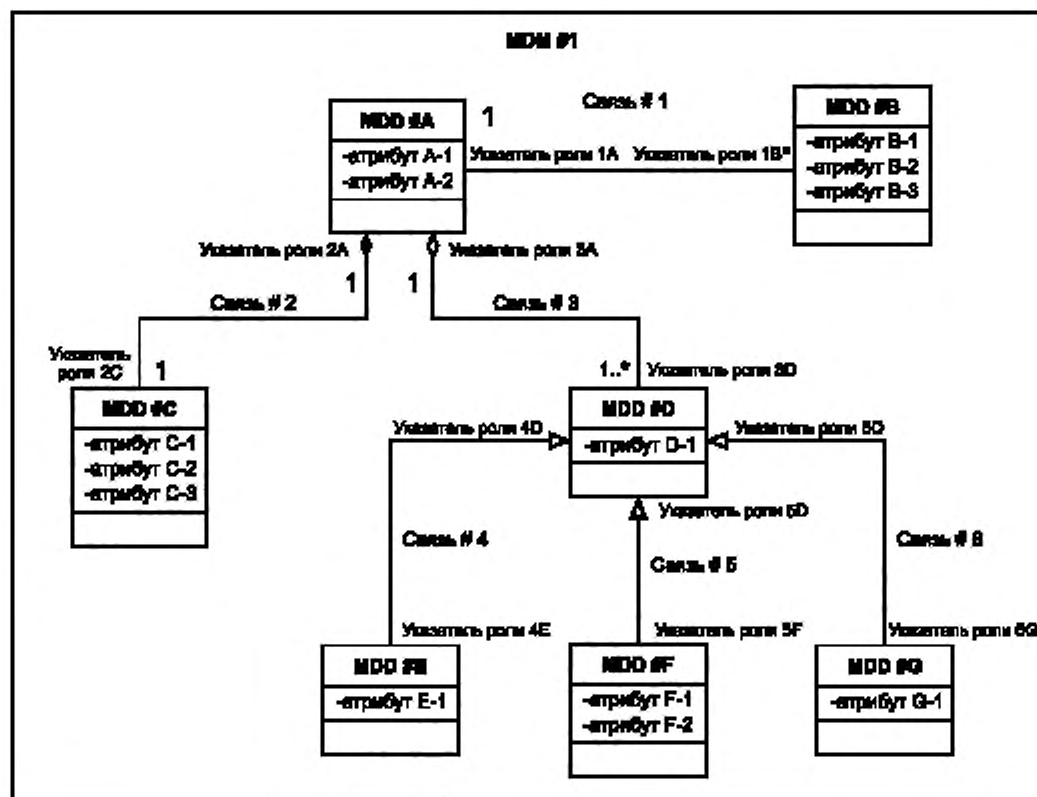
Рисунок 4 — Пример структуры MDM-модели
