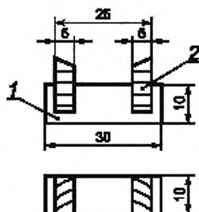
1 — металлическая оправка; 2 — образец из МД
