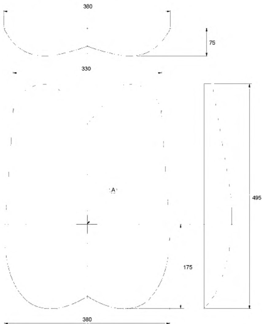
А — точка приложения нагрузки Рисунок 101 — Деревянный брусок
