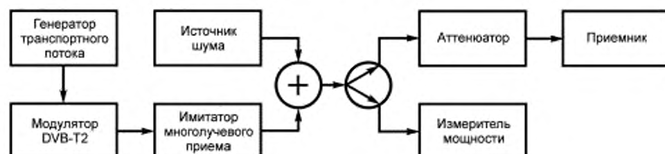
Рисунок 2 — Схема проверки 2
