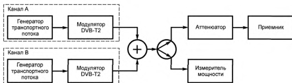
Рисунок 3 — Схема проверки 3
