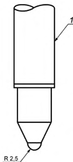
1 — нагрузочный шток
