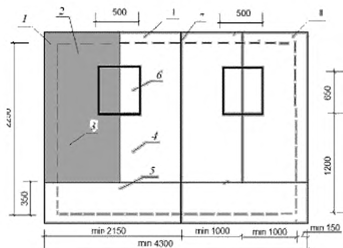
Рисунок 2 – Испытуемый фрагмент СФТК с двумя видами декоративно-защитного слоя
