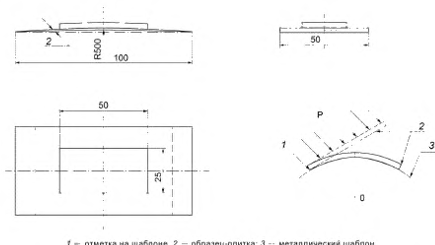
Рисунок 1 — Схема испытания на трещиностойкость
