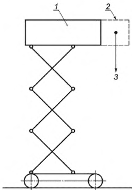
1 — основная рабочая платформа; 2 — платформа удлинения (полностью выдвинутое положение); 3 — номинальная нагрузка, т
