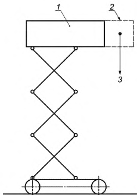
1 — основная рабочая платформа; 2 — платформа удлинения (полностью выдвинутая); 3 — номинальная нагрузка. m . Номинальная нагрузка определяется выражением (см. также 4.2.1):
