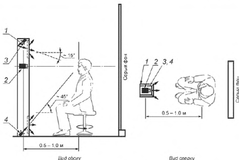
1 — консоль регистрации; 2 — камера; 3 — верхний осветитель; 4 — нижний осветитель
