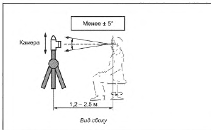
Рисунок С.2 — Рекомендации для взаиморасположения камеры и субъекта
