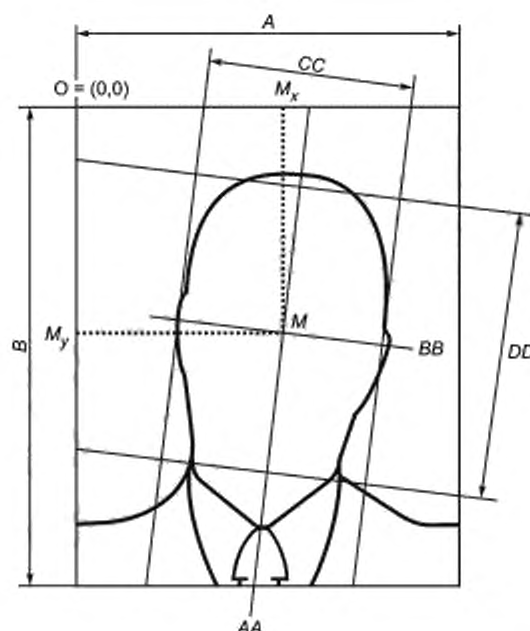
Рисунок 14 — Геометрические характеристики изображения лица полного фронтального типа
