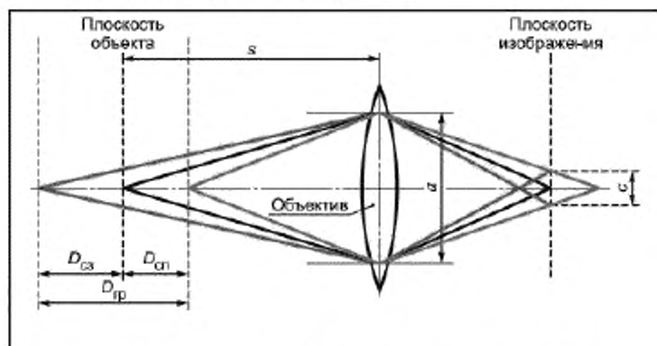
Рисунок С.1 — Параметры для вычисления глубины поля
